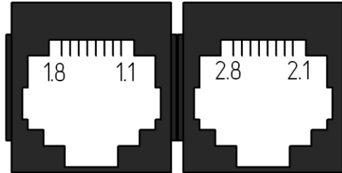
Рисунок 3 – Расположение сигнальных линий разъёма RJ45
