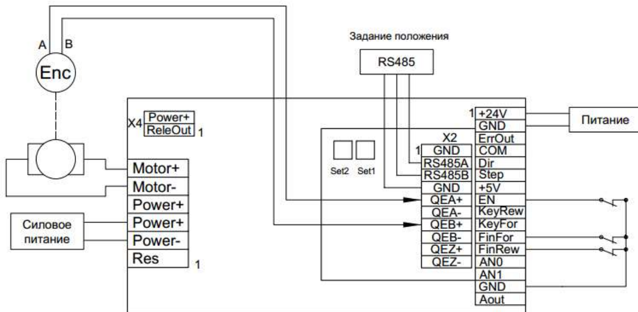
Рис. 29 – Управление угловым положением вала двигателя с обратной связью по квадратурному энкодеру. Задание кривой разгон-скорость-торможение с возможностью изменения параметров в процессе отработки
