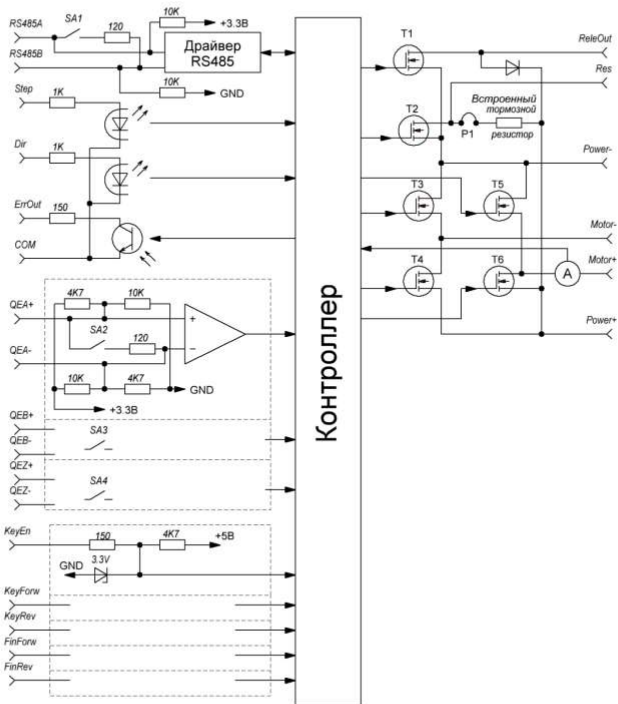
Рис. 3 – Схема входов и выходов блока управления AWD50
