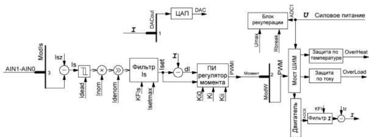
Рис. 22 – Структурная схема режима 5
