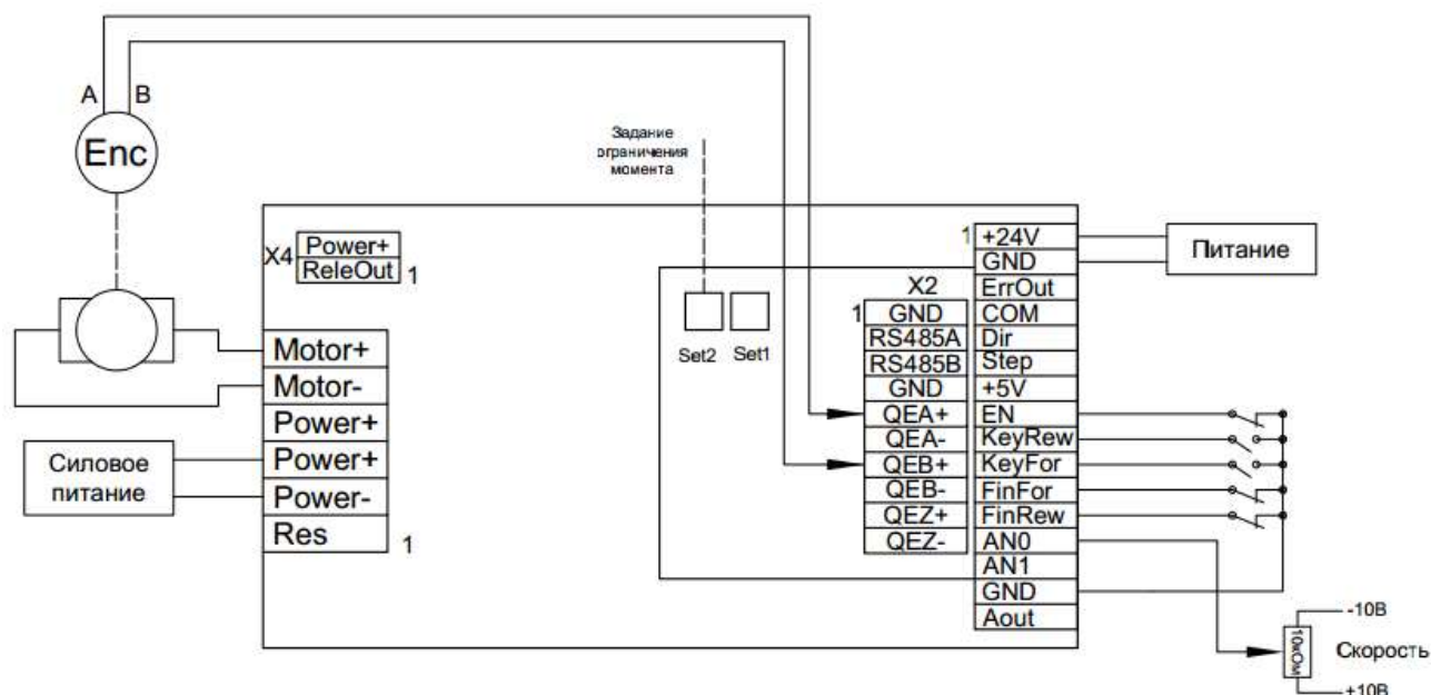
Рис. 16 – Управление скоростью вращения и ограничением момента коллекторного двигателя с обратной связью по квадратурному энкодеру
