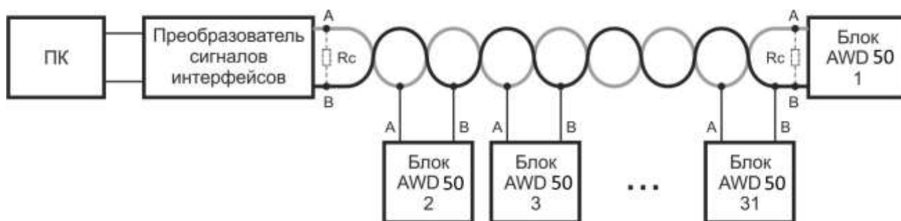
Рис. 7 – Пример подключения блока AWD50 к сети RS485
