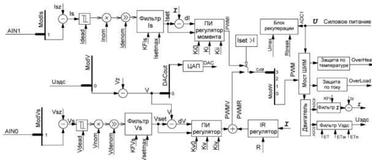
Рис. 26 – Структурная схема режима 7
