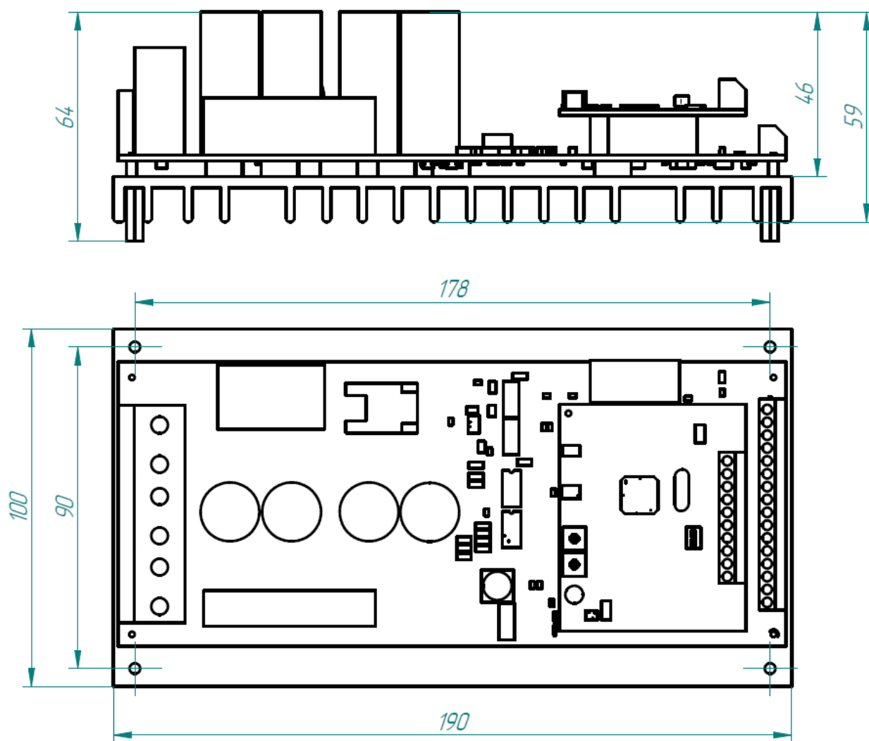
Рис. 1 – Габаритные размеры платы AWD50
