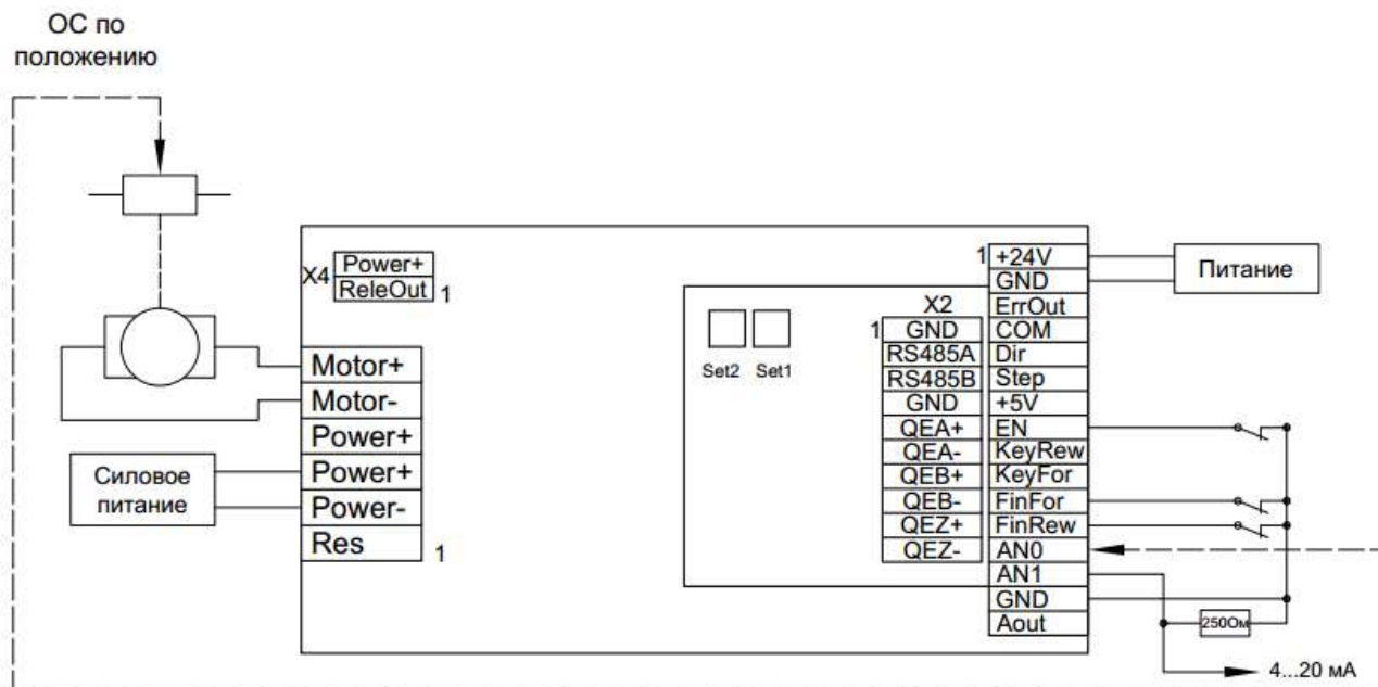
Рис. 20 – Управление положением исполнительного механизма с обратной связью по потенциометрическому датчику и аналоговым заданием. Управление с помощью токовой петли 4-20мА
