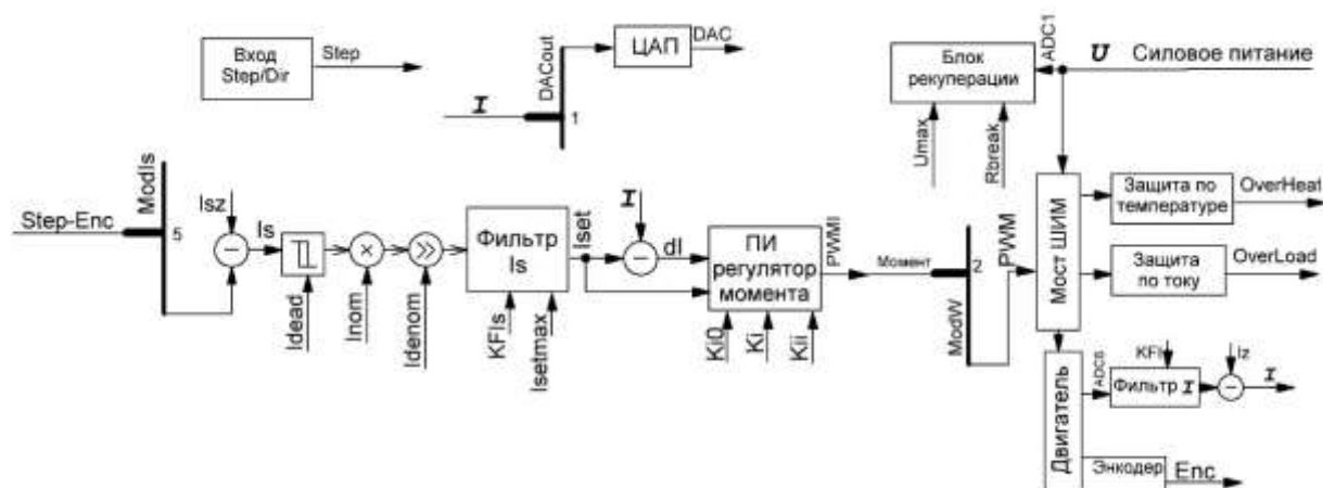
Рис. 28 – Структурная схема режима 8
