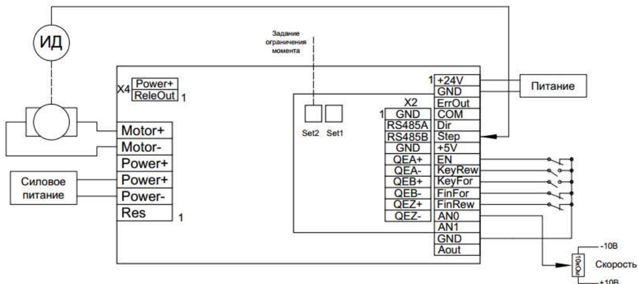
Рис. 18– Управление скоростью вращения и ограничением момента коллекторного двигателя с обратной связью по импульсному датчику
