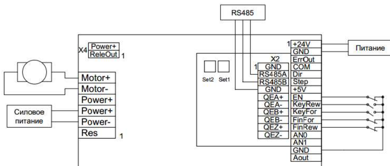
Рис. 25 – Управление механизмами без концевых выключателей с остановкой по переходу в режим стабилизации момента
