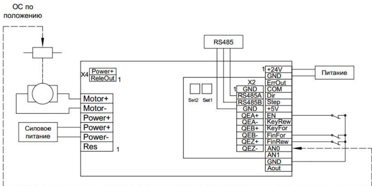
Рис. 23 – Управление положением исполнительного механизма с обратной связью по потенциометрическому датчику и заданием по RS485
