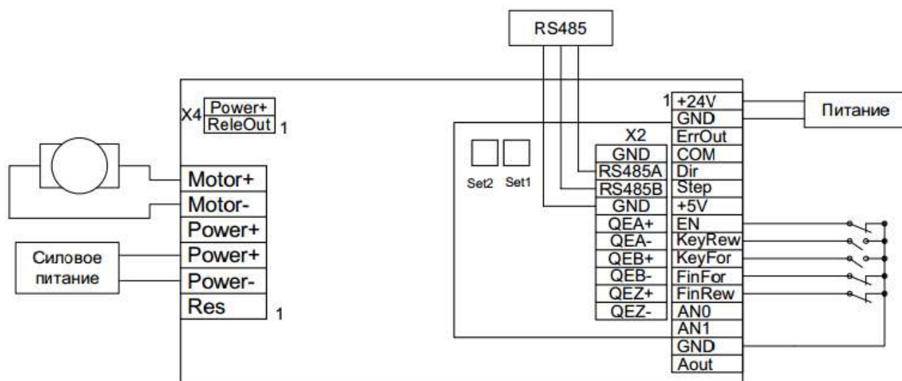
Рис. 12 – Управление скоростью вращения и ограничением момента коллекторного двигателя с постоянными магнитами или независимым возбуждением без дополнительных датчиков по RS485
