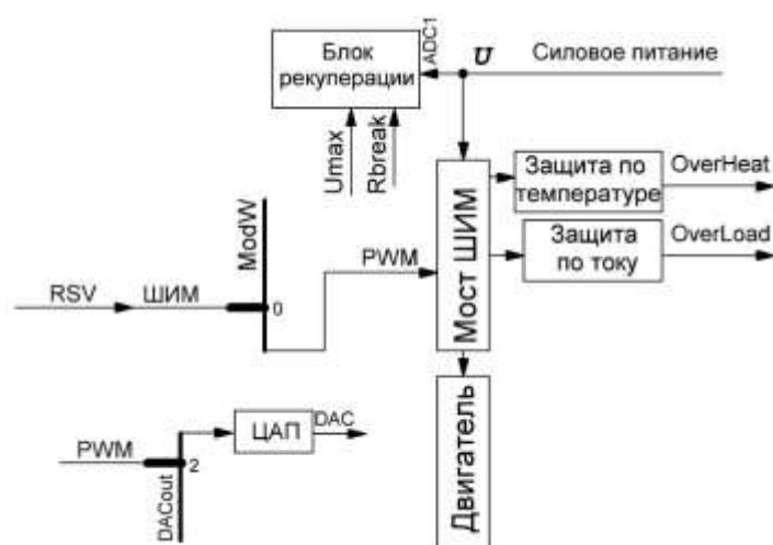
Рис. 33 – Структурная схема режима 11
