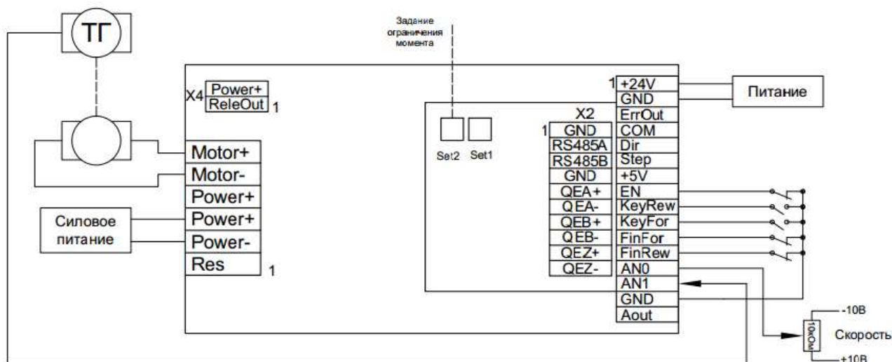
Рис. 14 – Управление скоростью вращения и ограничением момента коллекторного двигателя с обратной связью по тахогенератору
