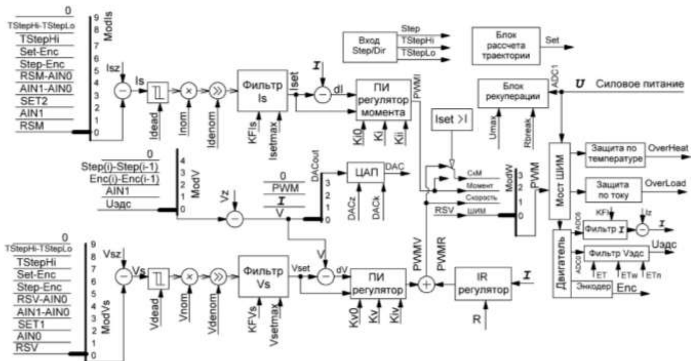
Рис. 4 - Структурная схема блока AWD50
