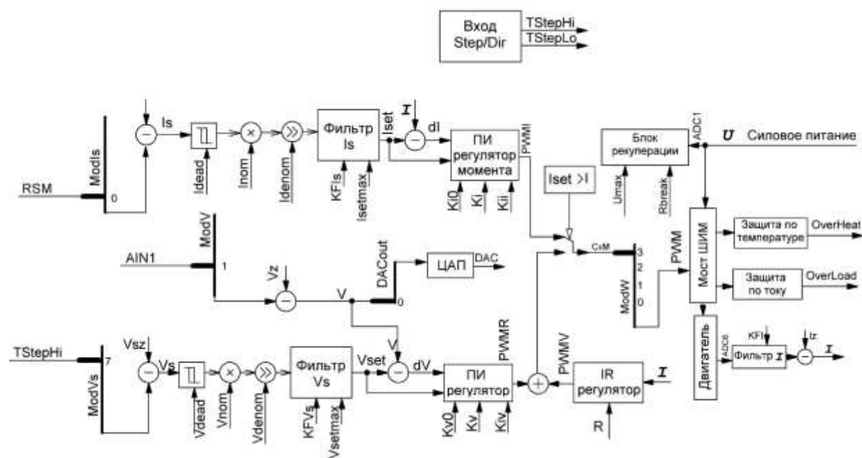
Рис. 35 – Структурная схема режима 12
