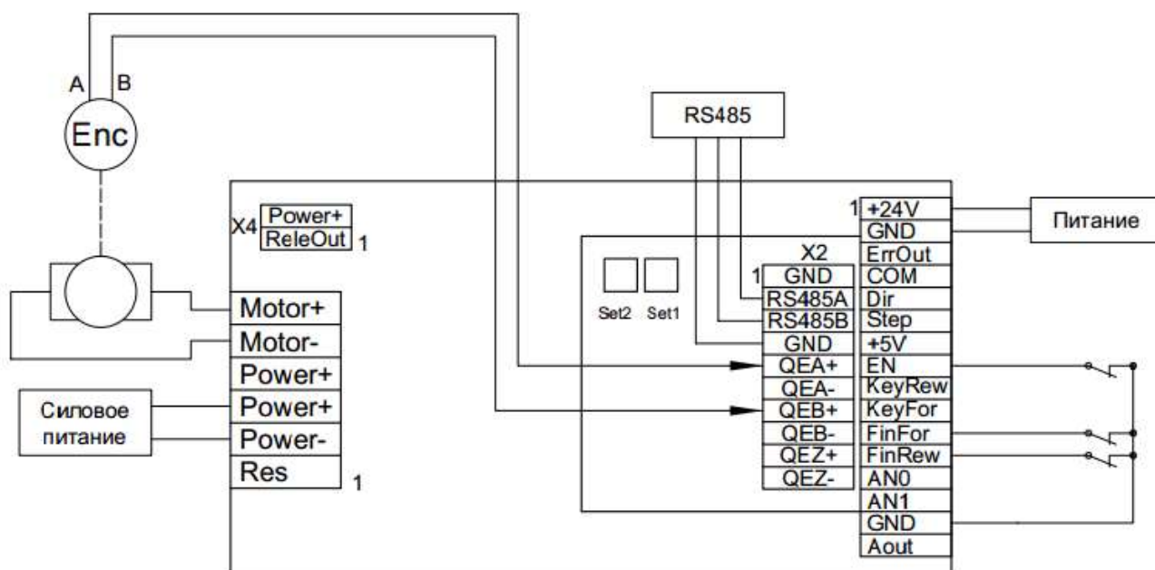
Рис. 31 – Реализация бесконечных колебаний между двумя точками любого механизма, снабжённого энкодером
