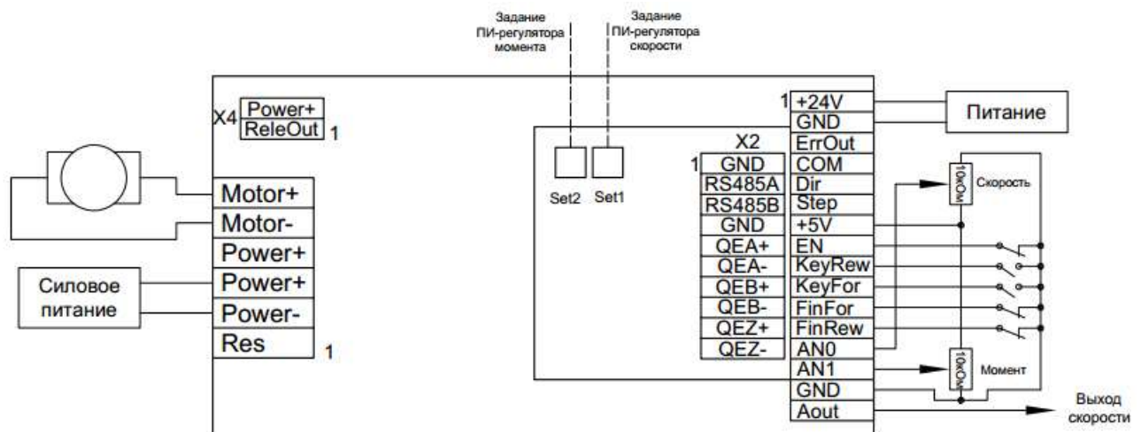
Рис. 8 – Управление скоростью вращения и ограничением момента коллекторного двигателя с постоянными магнитами или независимым возбуждением без дополнительных датчиков внешними аналоговыми сигналами
