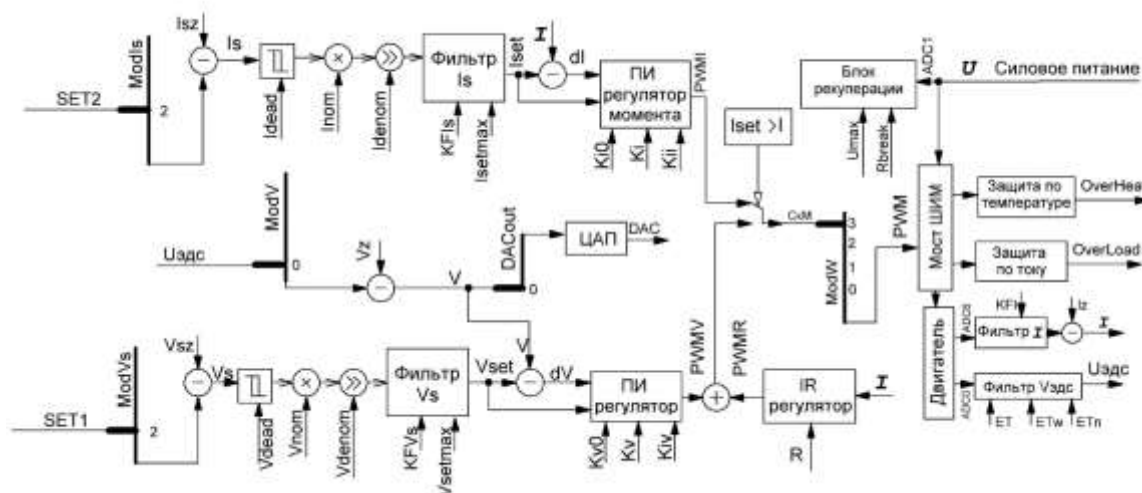
Рис. 11 – Структурная схема режима 16
