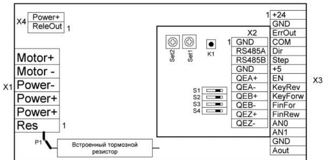
Рис. 6 – Расположение разъёмов блока управления
