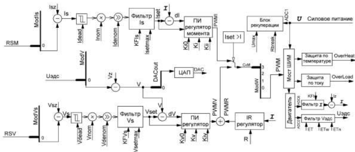
Рис. 13 – Структурная схема режима 1в
