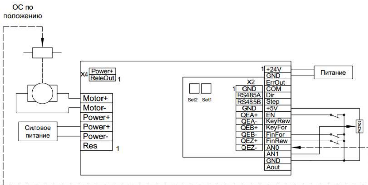
Рис. 21 – Управление положением исполнительного механизма с обратной связью по потенциометрическому датчику и аналоговым заданием. Управление с помощью разности между входами AN1 и AN0
