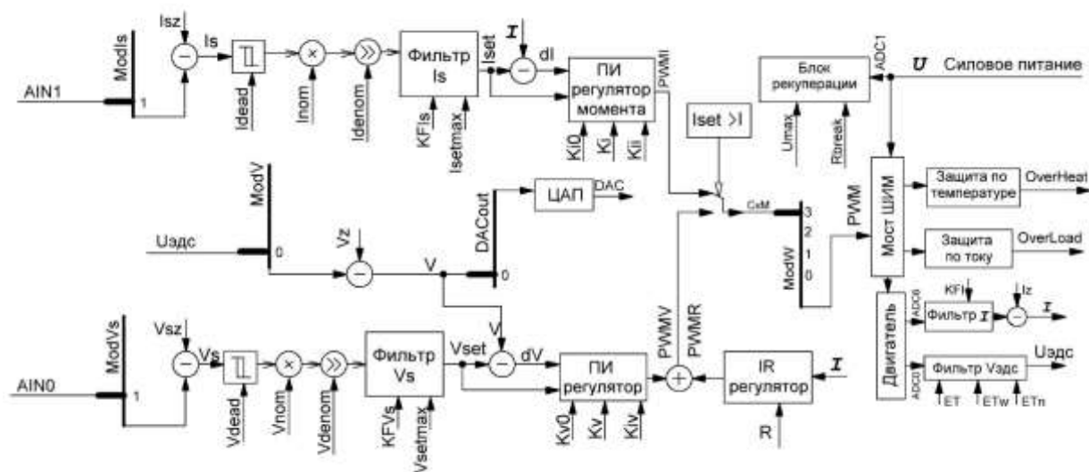
Рис. 9 – Структурная схема режима 1а
