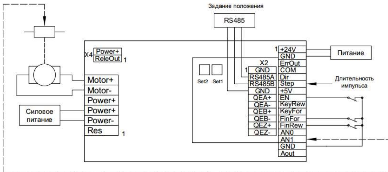
Рис. 34 – Управление углом поворота вала по сигналу PWM (аналог сервомашинки)
