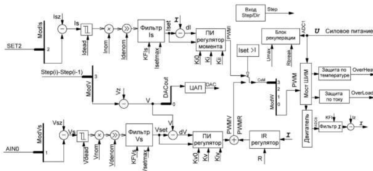
Рис. 19 – Структурная схема режима 4
