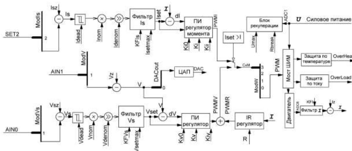
Рис. 15 – Структурная схема режима 2
