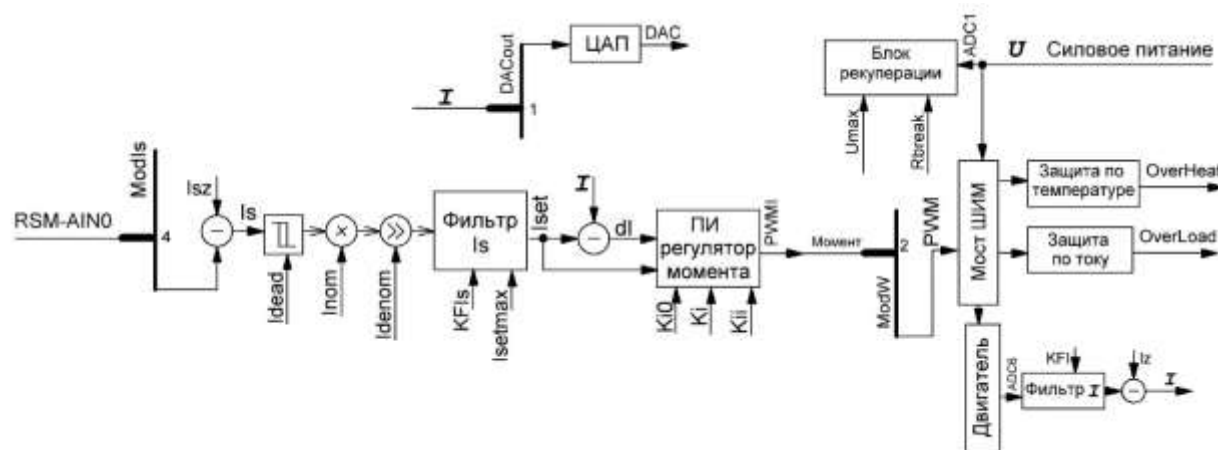
Рис. 24 – Структурная схема режима 6
