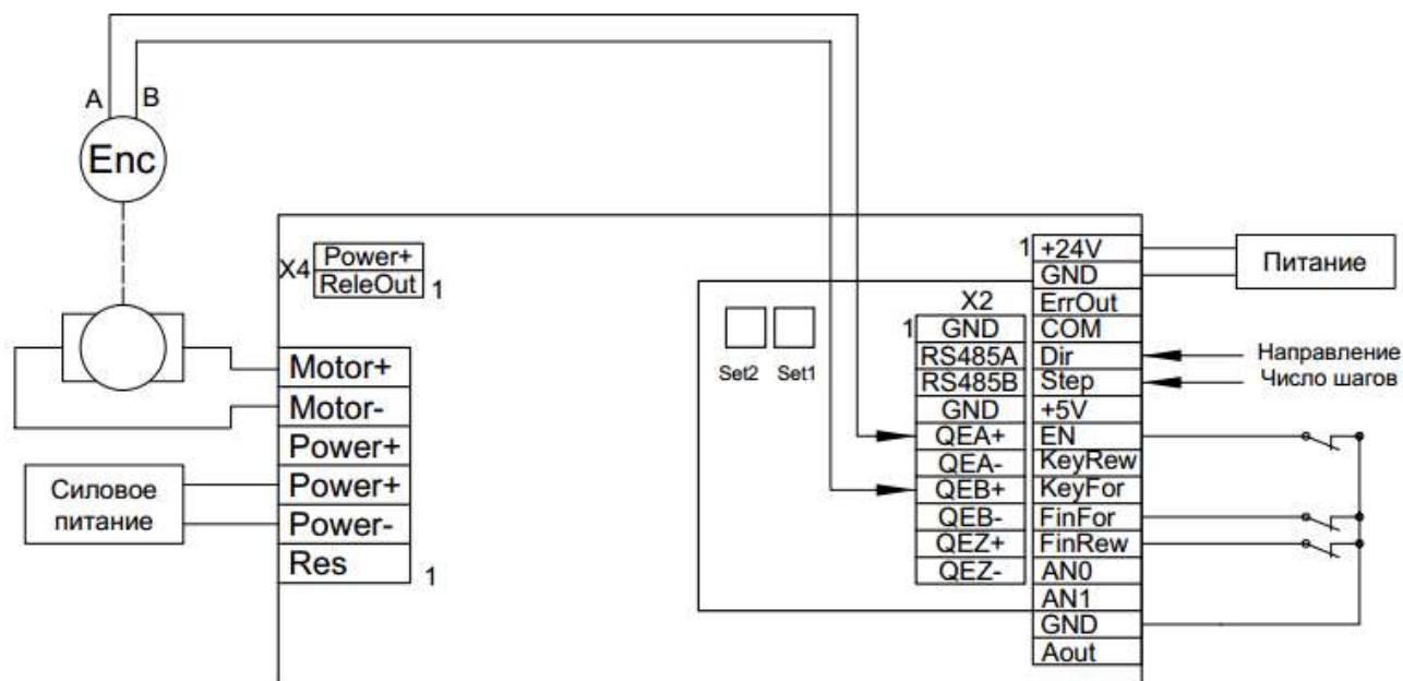
Рис. 27 – Реализация режима "шагового двигателя" с управлением положением входом Step/Dir и обратной связью по квадратурному энкодеру
