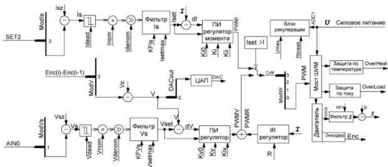
Рис. 17 – Структурная схема режима 3
