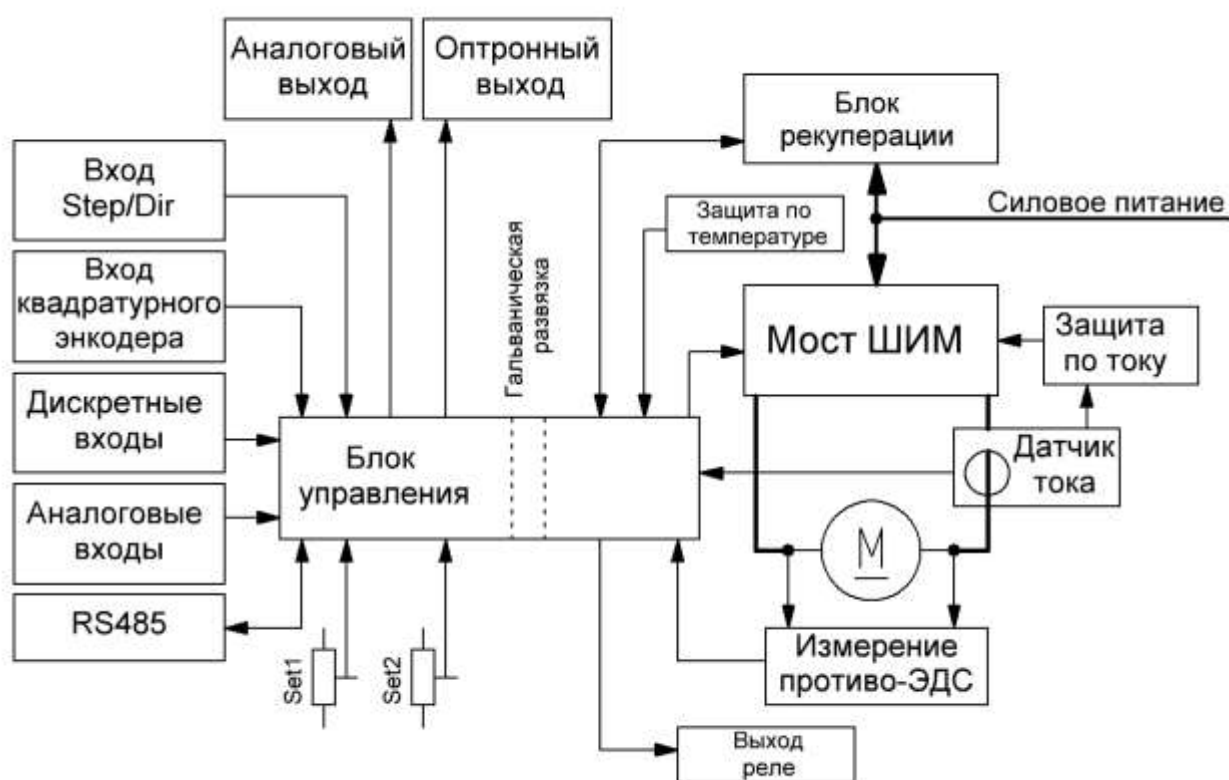
Рис. 2 – Функциональная схема блока управления AWD50
