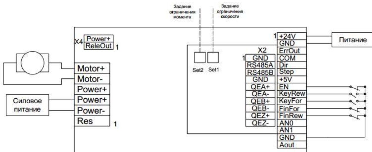
Рис. 10 – Управление скоростью вращения и ограничением момента коллекторного двигателя с постоянными магнитами или независимым возбуждением без дополнительных датчиков.
