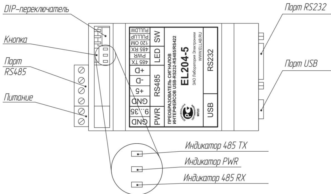
Рисунок 2 – Расположение разъёмов и индикации
