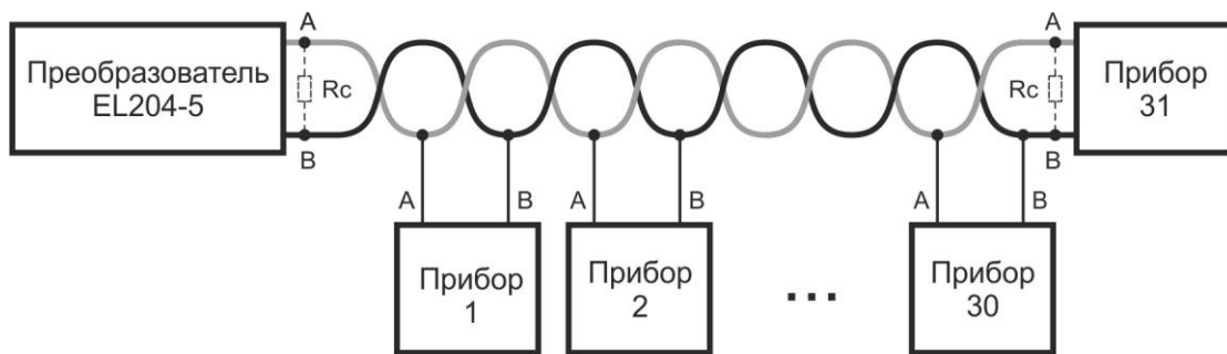
Рисунок 9 – Схема подключения преобразователя к сети RS485
