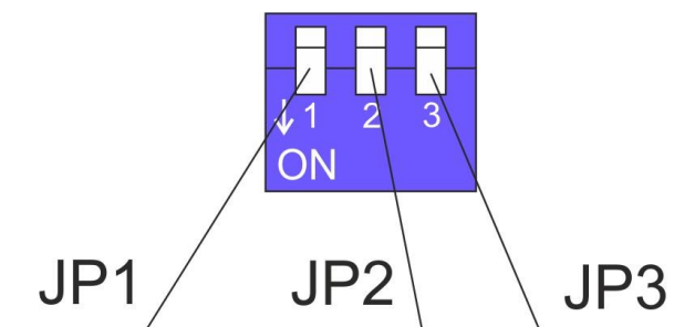
Рисунок 4 – настроечный DIP-переключатель порта интерфейса RS485
