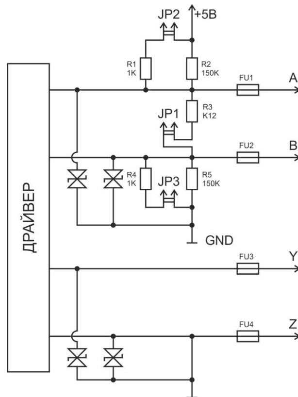
Рисунок 5 – Схема подключения драйвера RS485
