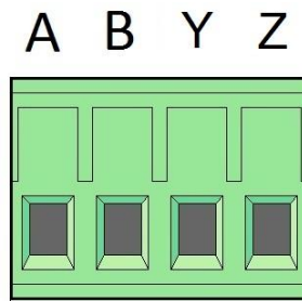
Рисунок 3 – Расположение сигнальных линий интерфейса RS485/RS422
