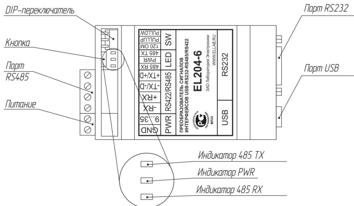
Рисунок 1 – Расположение разъёмов и индикации
