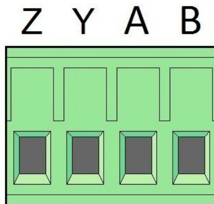
Рисунок 3 – Расположение сигнальных линий интерфейса RS485/RS422 на клеммной колодке переходника
