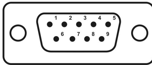
Рисунок 2 – Расположение сигнальных линий порта интерфейсов RS232/RS485/RS422 на разъёме DB9-F
