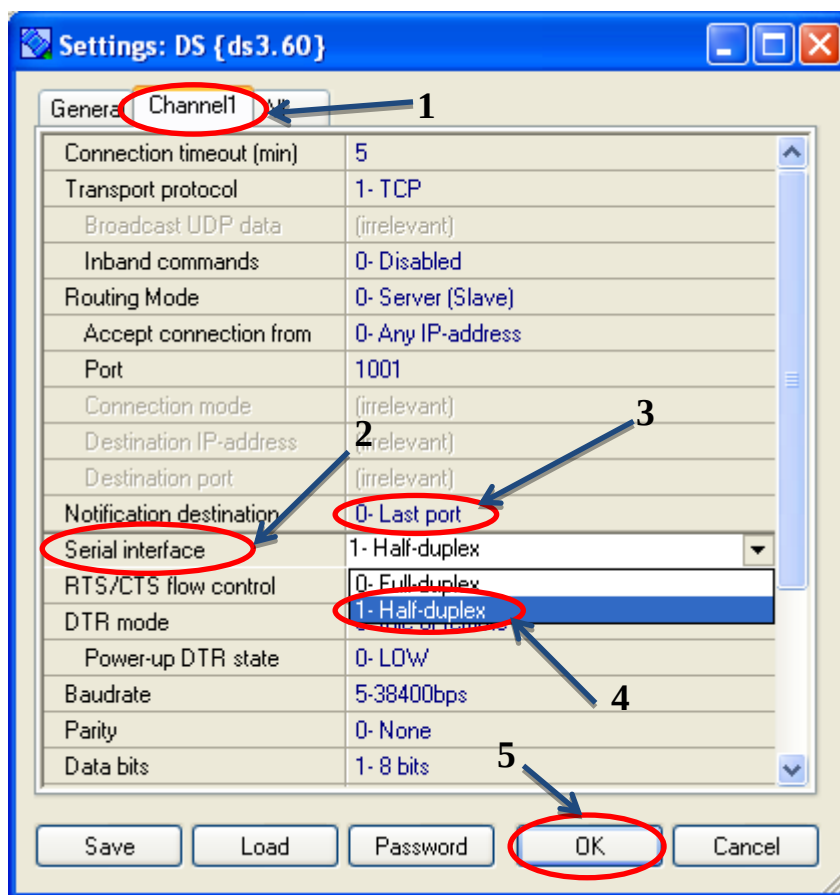
Рисунок 18 – Окно настроек Tibbo DS Manger
