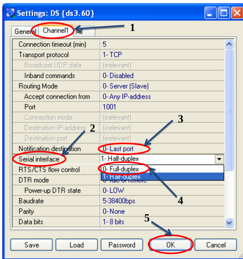
Рисунок 19 – Окно настроек Tibbo DS Manger
