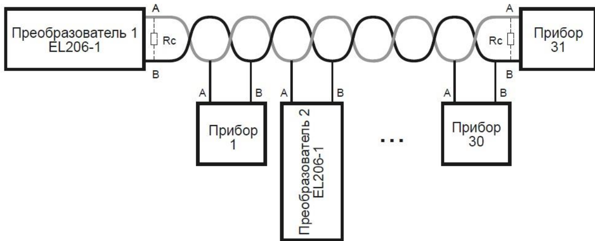
Рисунок 5 – Схема подключения преобразователя к сети RS485
