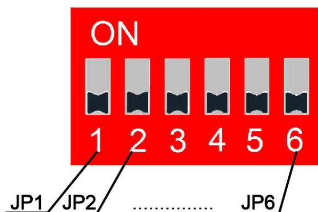
Рисунок 4 – Настроечный DIP-переключатель порта интерфейсов RS232/RS485/RS422
