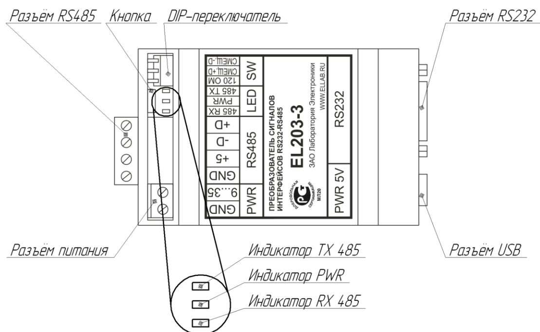
Рисунок 2 – Расположение разъёмов и индикации
